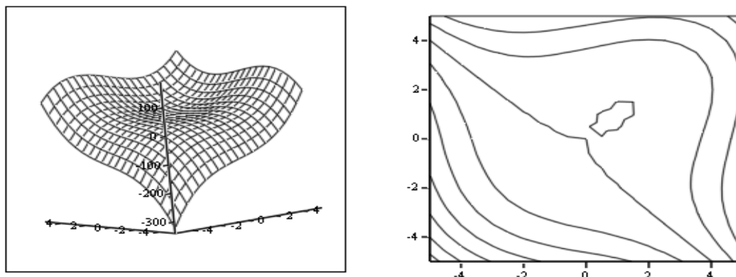
Рис.2. Графік функції C(x, y) = x^3 + y^3 - 3xy та її лінії рівня
