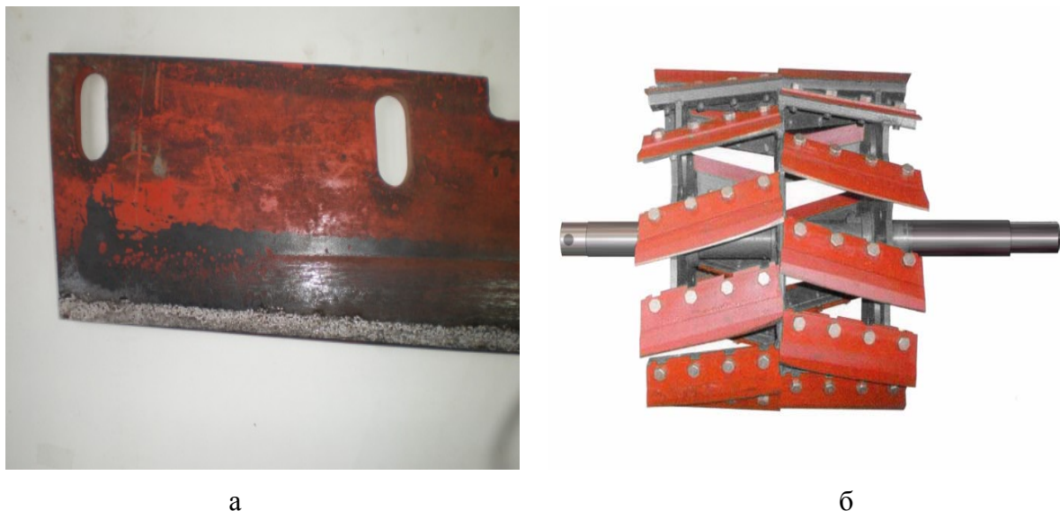
Рисунок 3 - Нож (а) измельчающего барабана (б) комбайна
