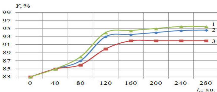
Рис. 1. Схожість отриманої зернової сировини в залежності від концентрації озону: 1 – при концентрації озону 10 \text{ мг/м}^3 ; 2 – при концентрації озону 15 \text{ мг/м}^3 ; 3 – при відсутності озону у складі сушильного агенту
