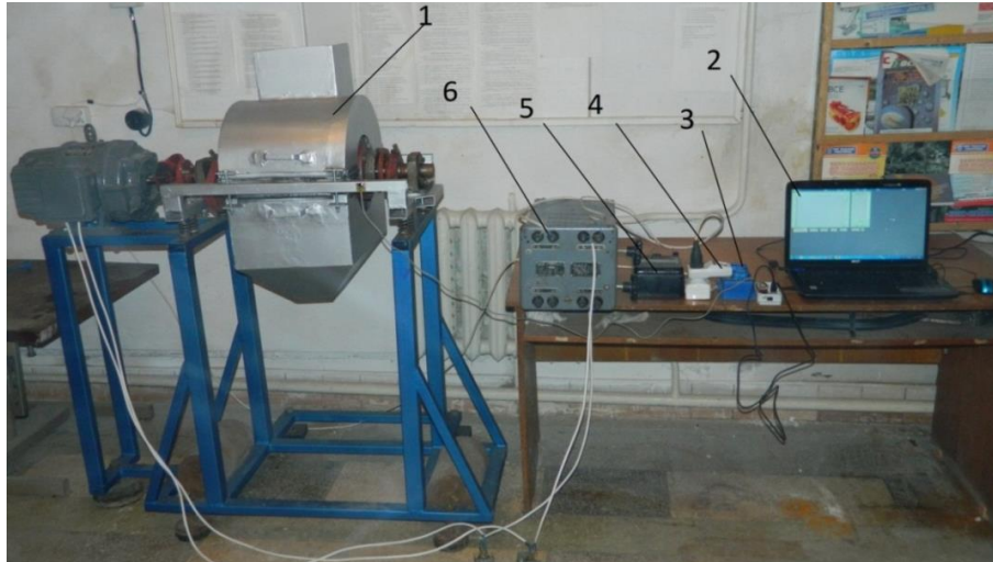
Рис. 2. Експериментальний стенд для дослідження розробленого обладнання: 1 – експериментально-дослідний зразок вібраційної дискової дробарки; 2 – персональний комп'ютер з програмним забезпеченням; 3 – вмикач; 4 – електронний ватметр EMF-1; 5 – дублюючий електромеханічний ватметр; 6 – лабораторний трансформатор АОСН-20-220-75.
