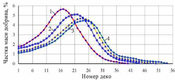
Рис. 4. Залежність розподілу суперфосфату гранульованого ТОН за напрямком розсівання за частоти обертання диска 800 об/хв. від кута його нахилу до горизонтальної площини: 1, 2, 3, 4 – кут нахилу диска до горизонтальної площини відповідно 0°, 10°, 20°, 30°
