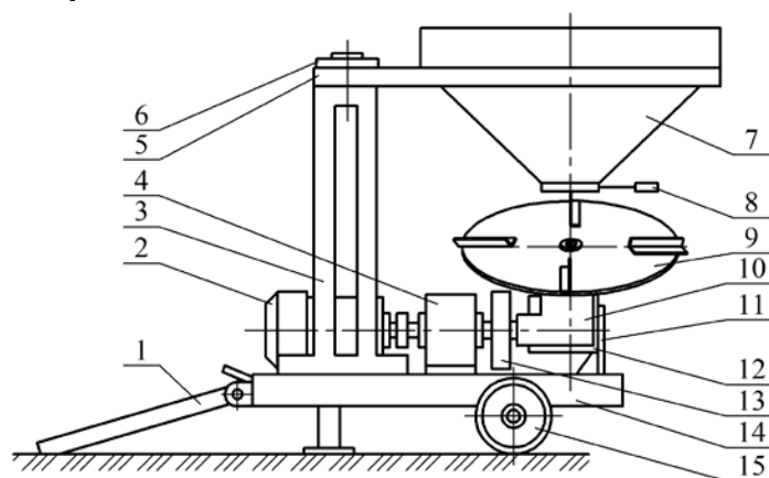
Рис. 1. Схема експериментальної установки: 1 – рукоять; 2 – електродвигун; 3, 5 – відповідно рухома та поворотна рами; 4 – ланцюговий варіатор; 6 – шарнір повороту рами; 7 – бункер; 8 – заслінка; 9 – ТОН; 10 – конічний редуктор; 11, 12 – кронштейни; 13 – обгінна муфта; 14 – основна рама; 15 – опорне колесо
