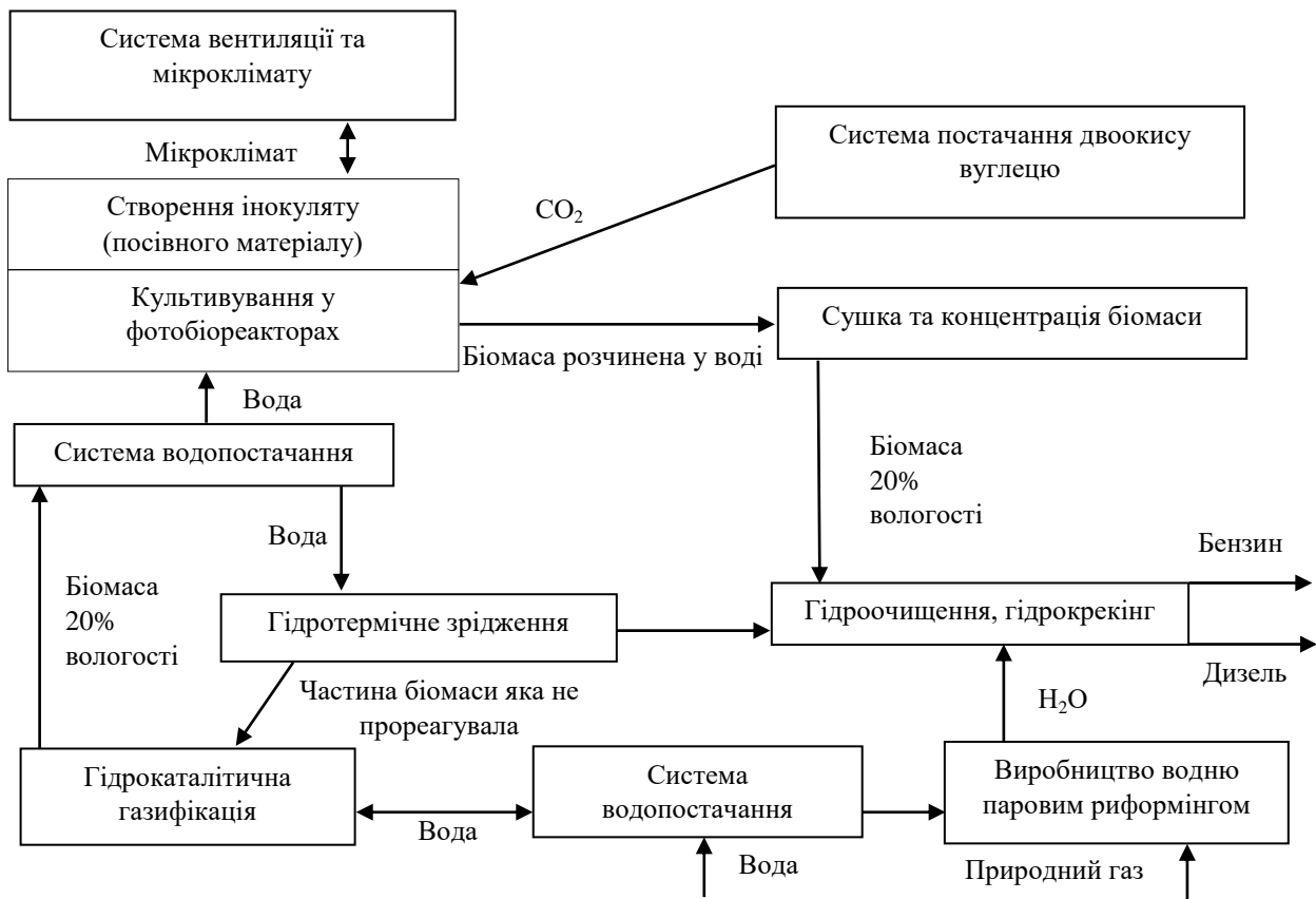
Рис. 3. Концептуальна схема технології отримання біодизелю із мікроводоростей
