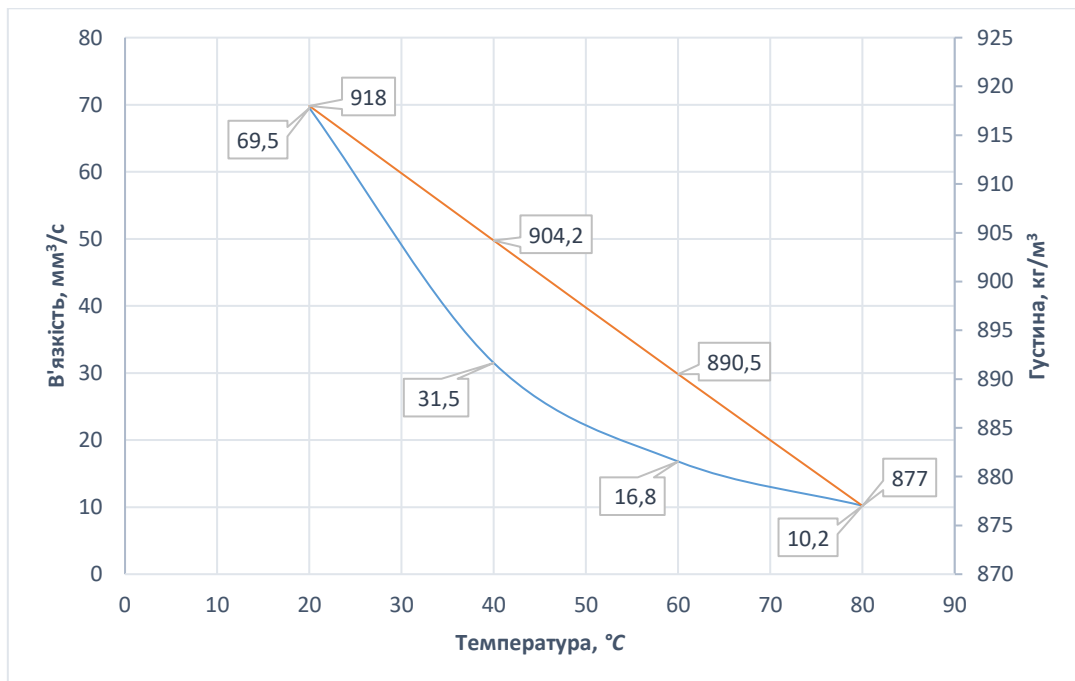
Рис. 7. Вплив температури на в'язкість та густину ріпакової олії
