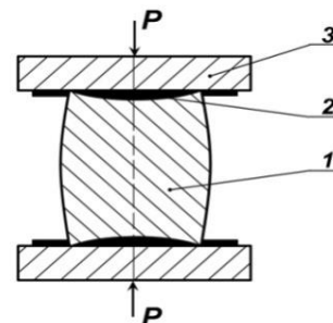
Рис. 1. Схема осадження суцільного циліндричного зразка із забезпеченням умов одноосного стиску: 1- зразок, 2-фольга, 3- інструмент
