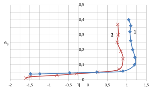
Рис. 6. Траєкторії шляхів деформування точки зовнішньої 1 та внутрішньої 2 вільних бічних поверхонь заготовки
