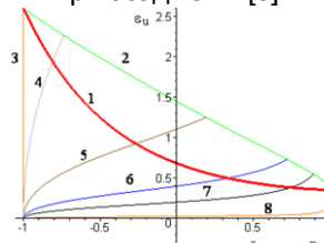
Рис. 4. Залежність граничного стану матеріалу від інтенсивності бочкоутворення при осадженні: 3-8 траєкторії деформування, де 3 – m=30; 4 – 2; 5 – 0,5; 6 – 0,18; 7 – 0,09; 8 – 0,01
