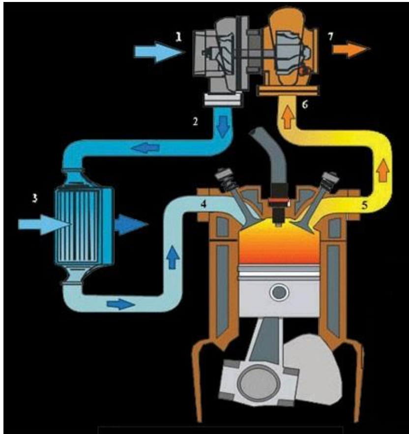
Рис. 1. Схема двигуна з наддуванням:
