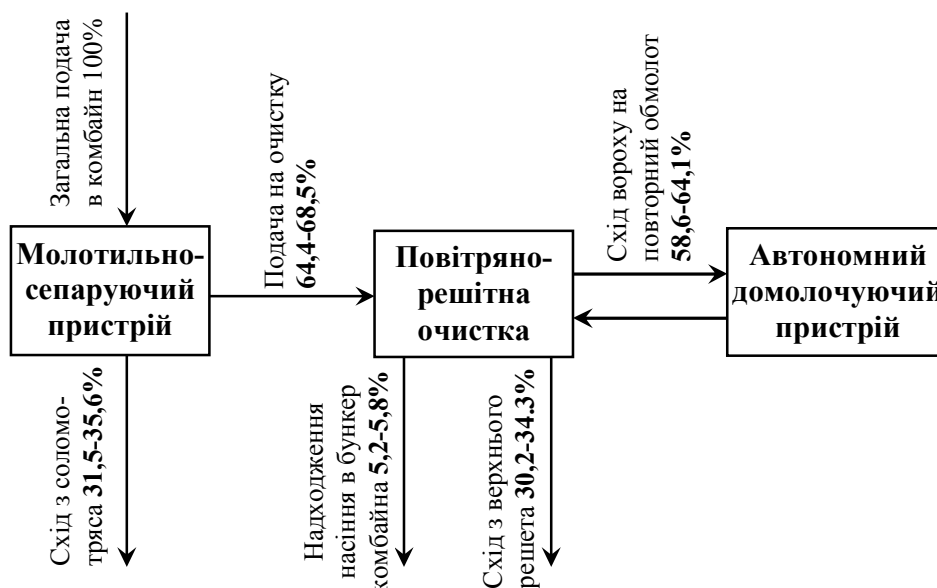
Рис. 1. Схема технологічних потоків в молотарках зернозбиральних комбайнів при збиранні насіння багаторічних бобових трав
